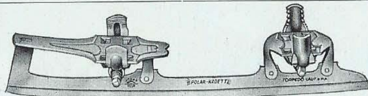
Kinderschlittschuh „Polar-Kadett“ mit Torpedo-Lauf DRP. Eine Nummer brauchbar für drei Centimetergrößen. Hergestellt in folgenden Größen
