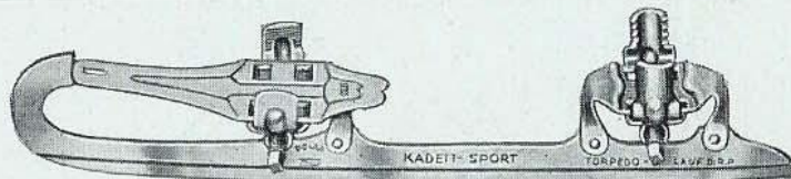
Jugendschlittschuh „Kadett-Sport“ mit Bogen u. Torpedo-Lauf DRP., sonst wie „Polar-Kadett“. Eine Nummer brauchbar für drei Centimetergrößen. Hergestellt in folgenden Größen
