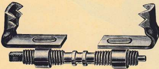
14 Zadní pár ztužidel se šroubem a matkami
